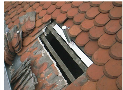
Stützenmontage
